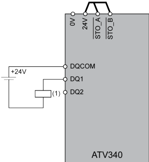
(1) relé o válvula
