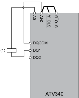
(1) relé o válvula
