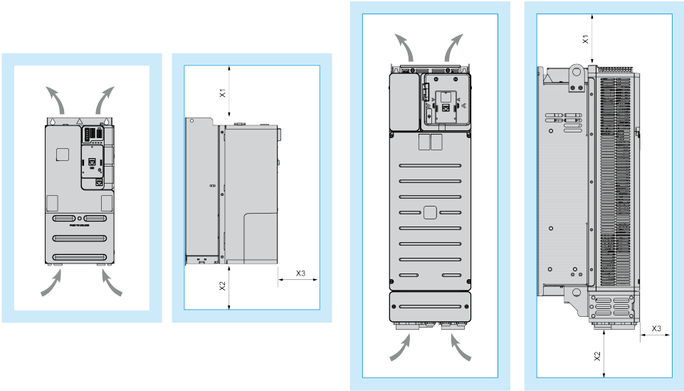
Separación mínima en relación con el tamaño del bastidor del variador
