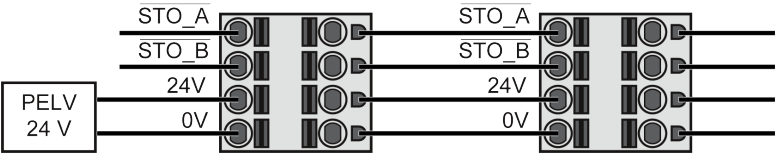
Conexión alternativa: cableado de variador a variador
