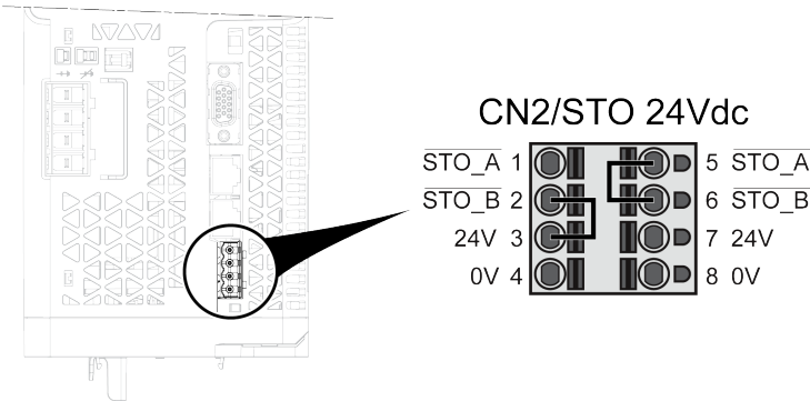
Conexión alternativa: cableado de variador a variador
